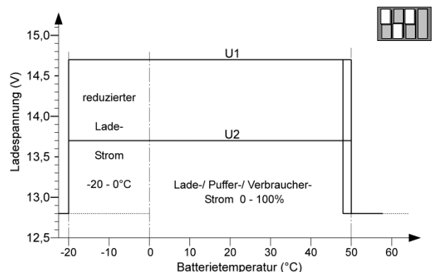
g) LiFePO4 14,7 V, nur für Sonderanwendung!
