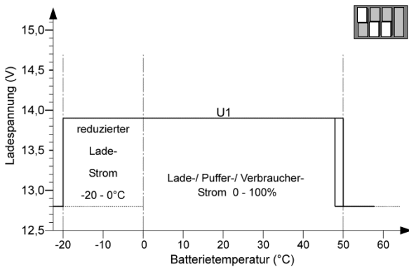
d) LiFePO4 13,9 V, Dometic „eStore“
