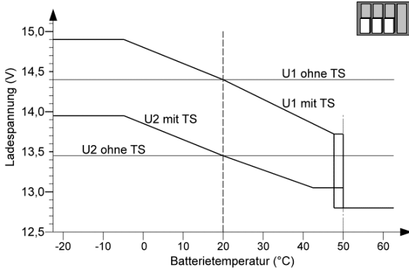
a) Blei „Lead Acid/AGM1“, Kennlinie IU1oU2
