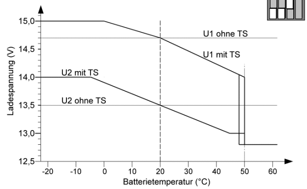
b) Blei „AGM2“, Kennlinie IU1oU2
