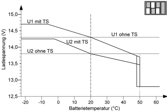
c) Blei „GEL“, Kennlinie IU1oU2
