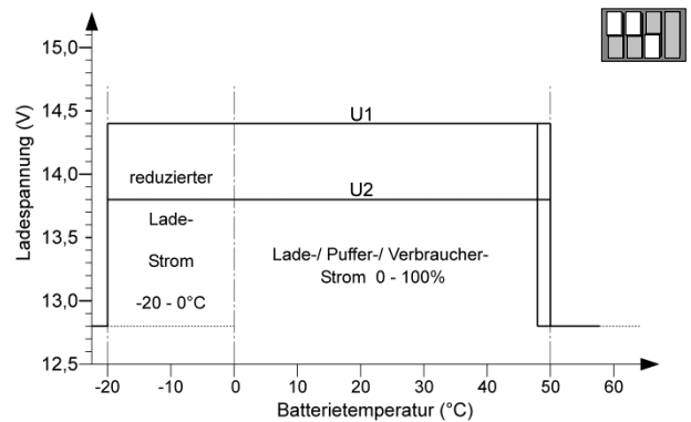
e) LiFePO4 14,4 V, Super B SB12VxxE, GNB SL12 xxxHC
